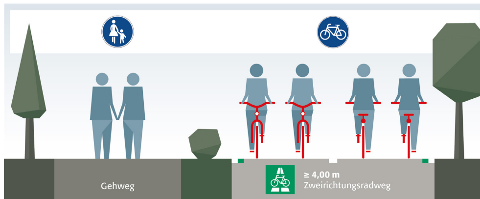
Abbildung 2: Musterquerschnitt RSV als selbstständiger Radweg im Zweirichtungsverkehr (eigene Darstellung)
