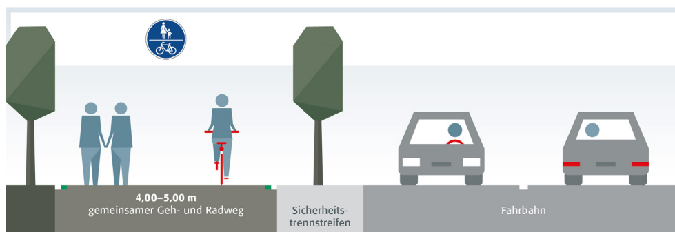
Abbildung 4: Musterquerschnitt RSV als gemeinsamer Rad-/Gehweg im Ein- und Zweirichtungsverkehr (eigene Darstellung)
