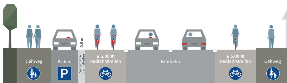
Abbildung 5: Musterquerschnitt RSV als Radfahrstreifen (eigene Darstellung)
