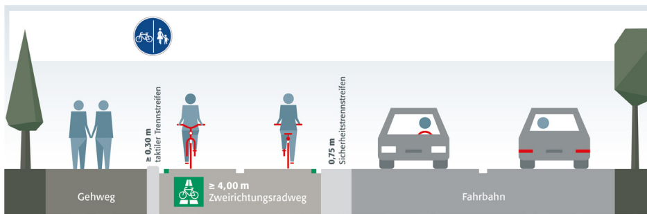
Abbildung 6: Musterquerschnitt RSV als getrennter Rad-/Gehweg im Zweirichtungsverkehr (eigene Darstellung)
