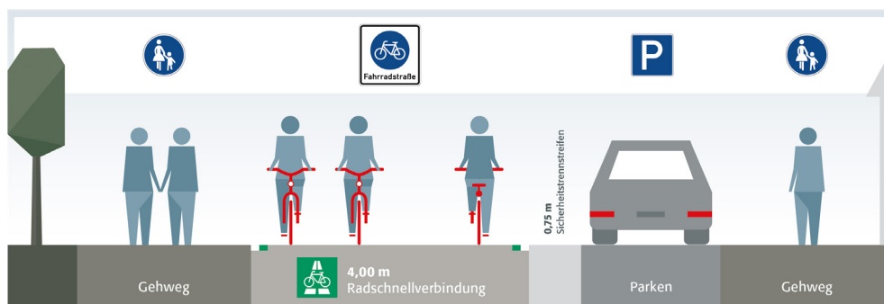
Abbildung 7: Musterquerschnitt RSV als Fahrradstraße (eigene Darstellung)
