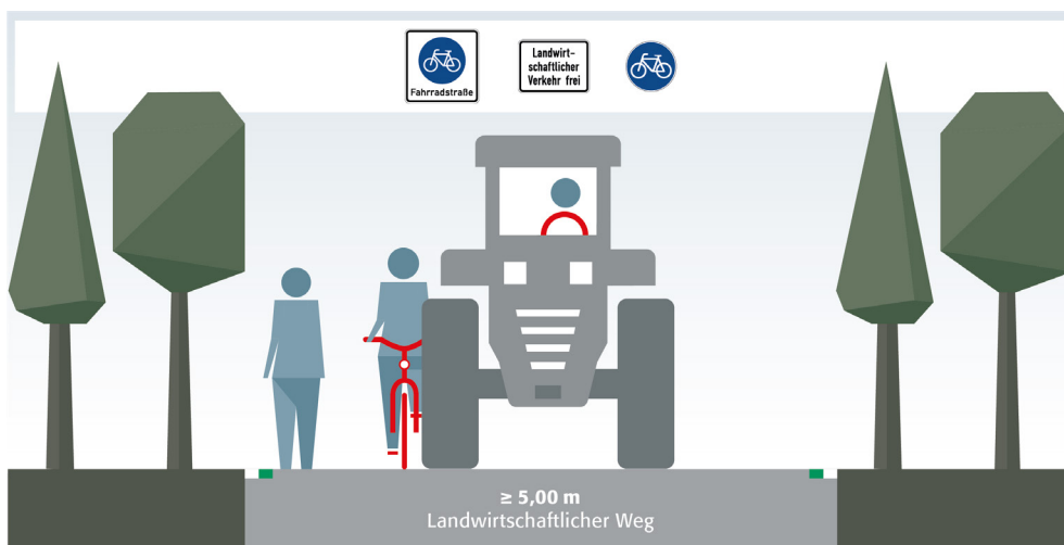
Abbildung 8: Musterquerschnitt RSV als Fahrradstraße außerorts mit freigegebenen land- und forstwirtschaftlichem Verkehr (eigene Darstellung)
